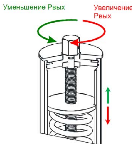
Рисунок 8 – Настройка выходного давления
