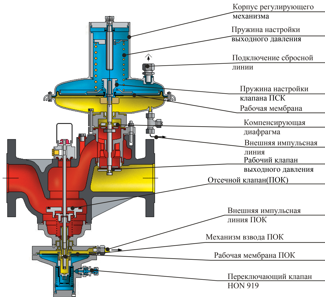
Рисунок 4 – Устройство регуляторов HON330 (Ду80, Ду100)
