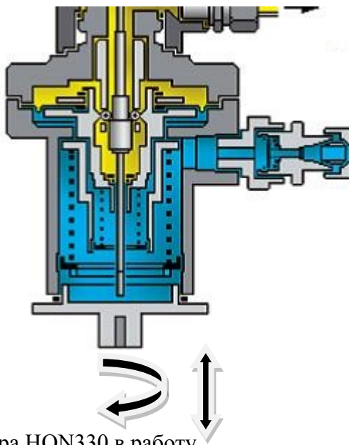
Рисунок 7 – Пуск регулятора HON330 в работу
