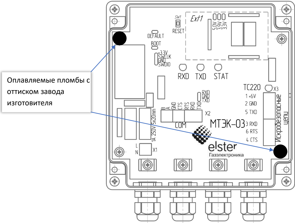
Рисунок 1 Схема пломбировки модуля МТЭК-03
